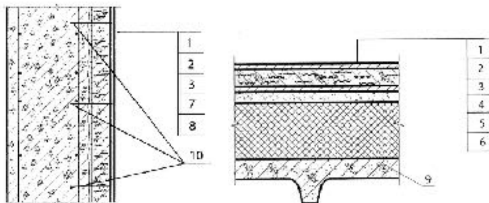
Рис.8.13. Примеры применения торкрет-фибробетонных покрытий в вертикальном (стена силоса – а) и горизонтальном (кровля – б) исполнениях
