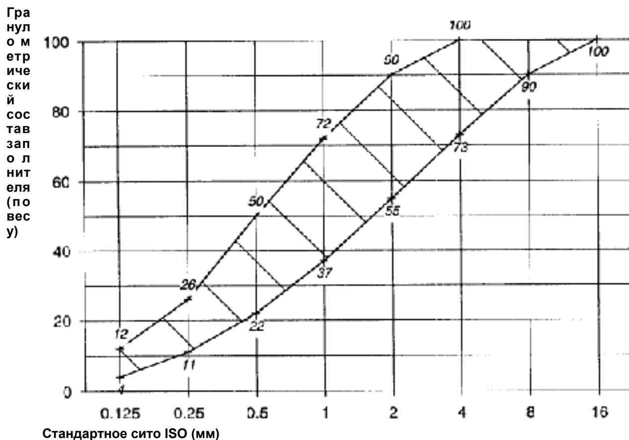
Рисунок 1. Требуемый гранулометрический состав песка
